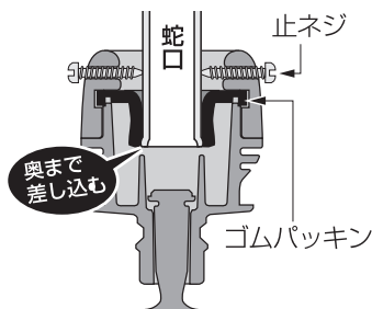
蛇口ニップル断面図
