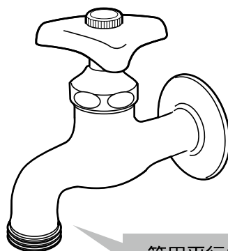
管用平行ネジ G3/4
