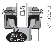
(蛇口ニップル断面図)
